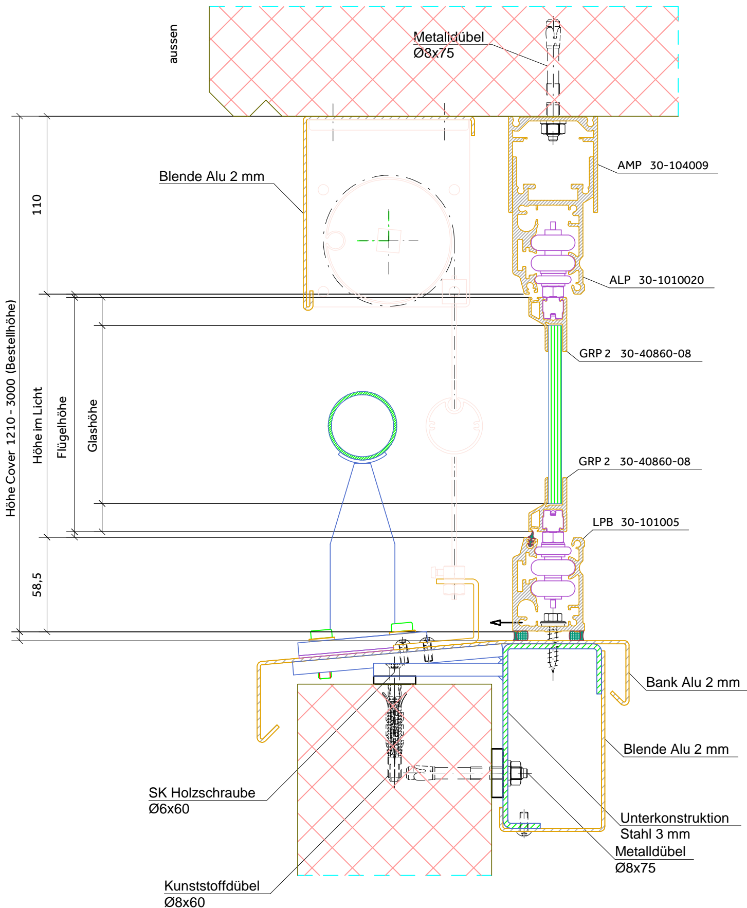
Detail Brüstung mit Aluminiumbank, Geländer und Store
