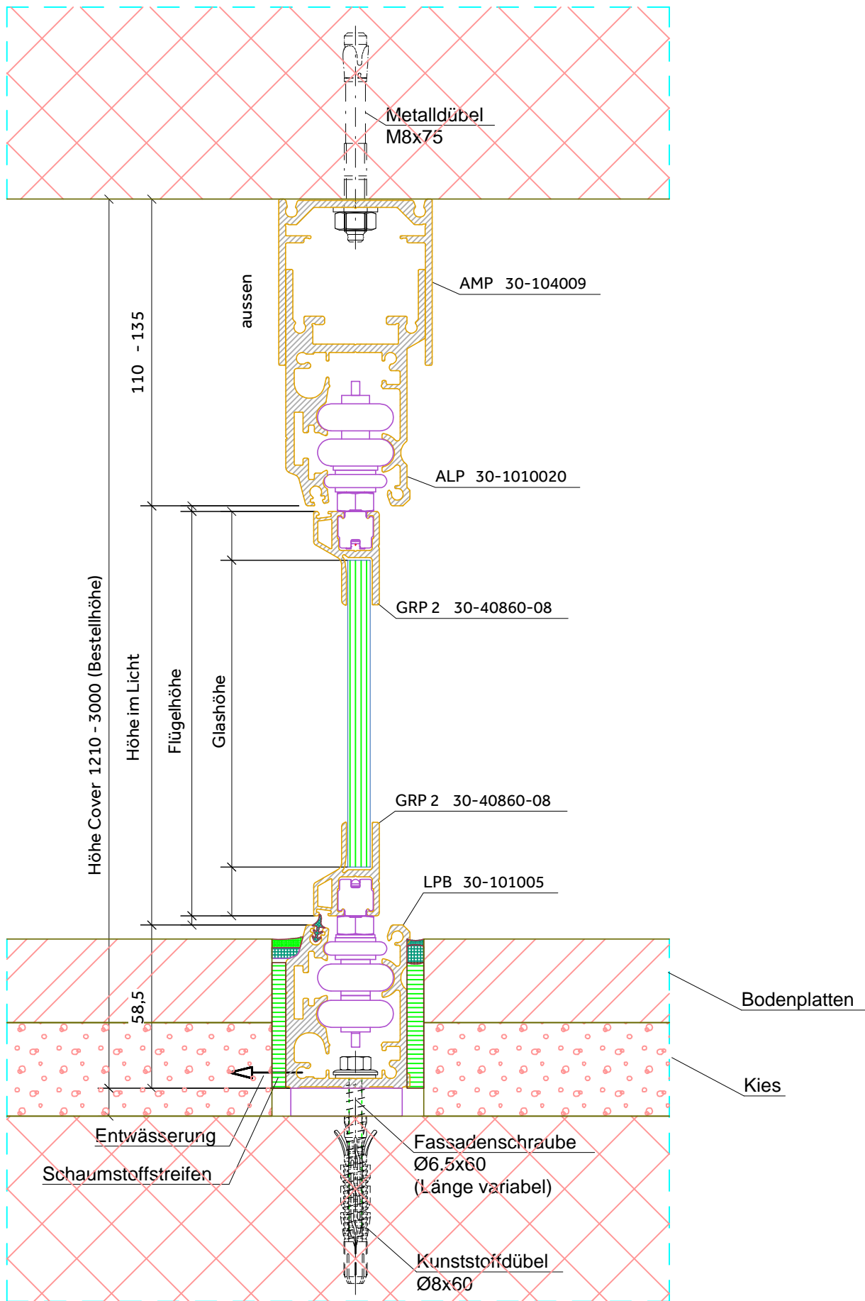
Bodendetail Schiene versenkt Entwässerung in Boden
