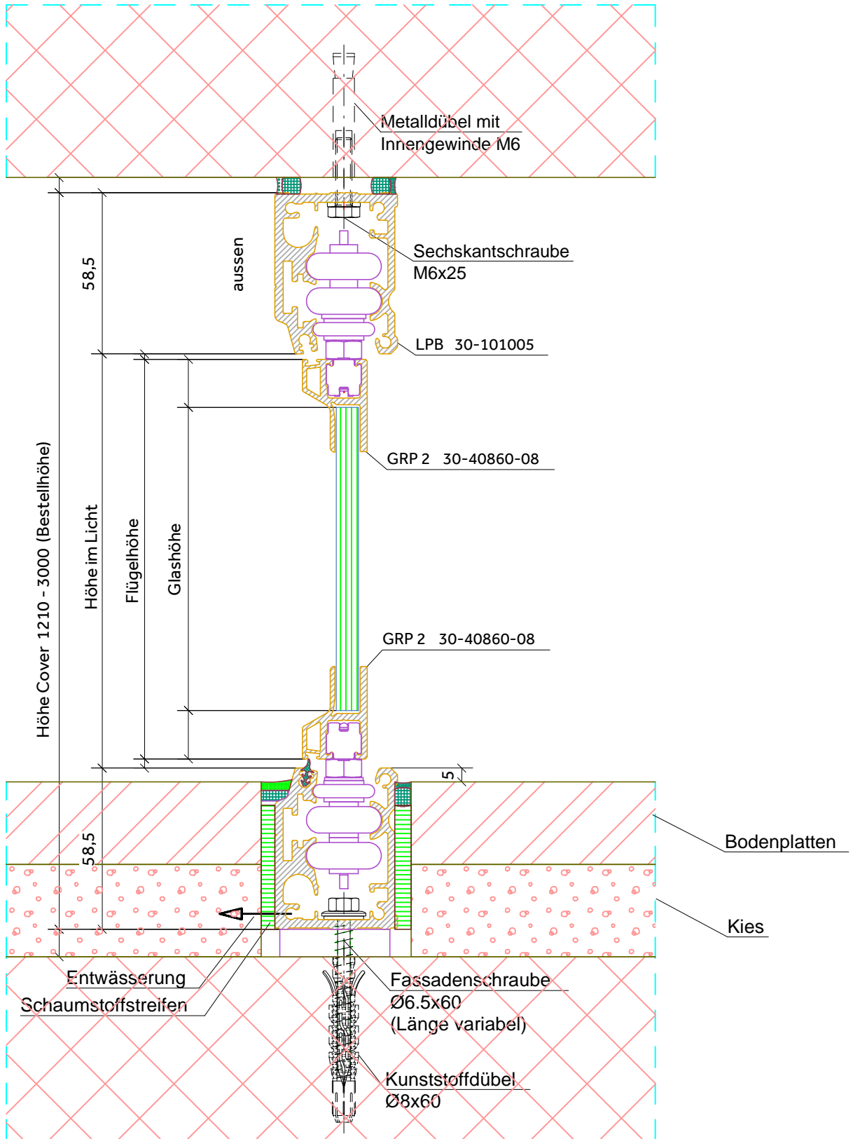
Bodendetail Schiene versenkt Entwässerung in Boden
